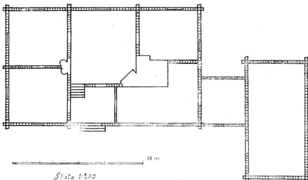
Planritning över boställsbyggnaden
